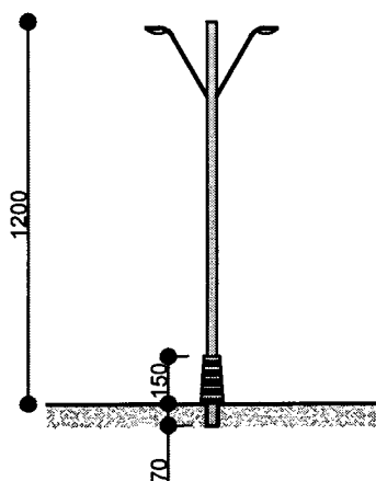
POSTE COM PROTEÇÃO APLICÁVEL AOS POSTES 07, 08 E 09
