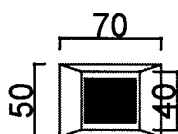
POSTE COM PROTEÇÃO APLICÁVEL AOS POSTES 07, 08 E 09
