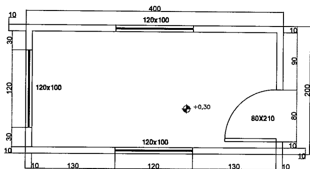
PLANTA GUARITA Escala: 1:10
