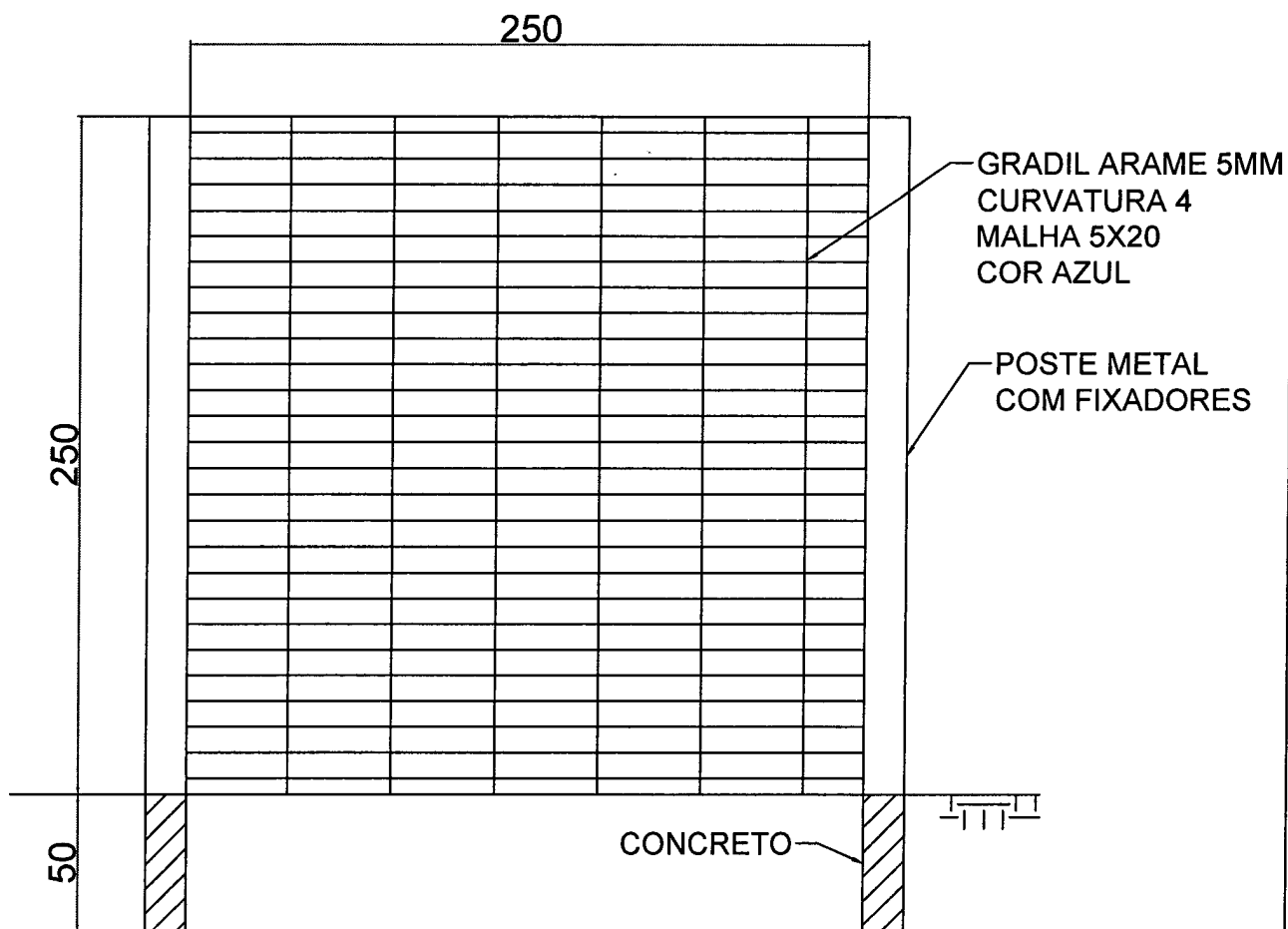
DETALHE GRADIL
