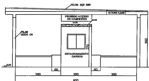
ELEVAÇÃO GUARITA FRENTE Escala: 1:25
