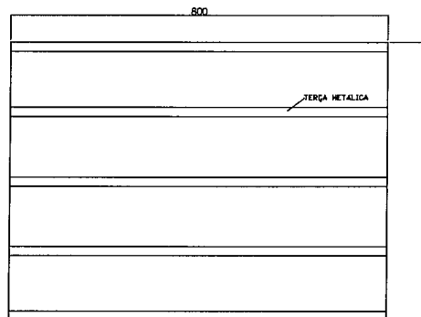
PROJEÇÃO COBERTURA Escala: 1:25
