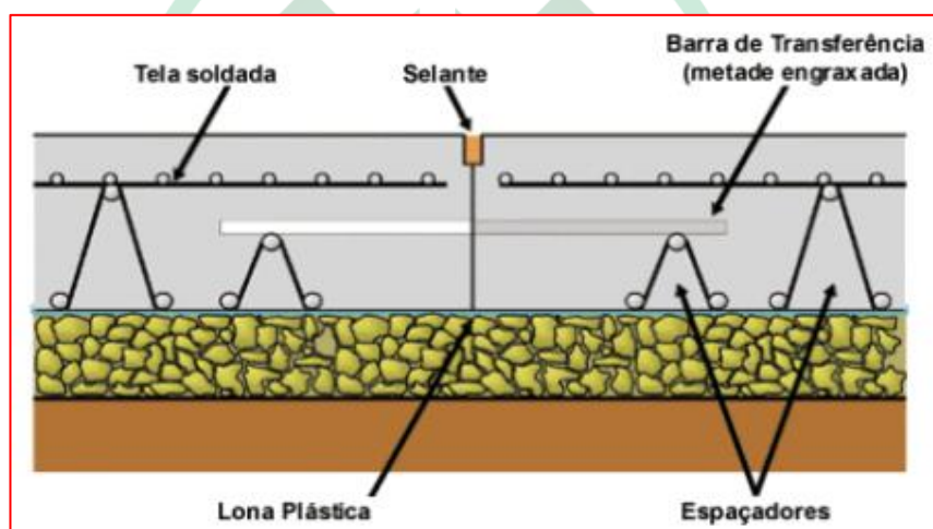
Figura 11 - Detalhe da seção transversal do piso industrial – Fonte: GOOGLE
