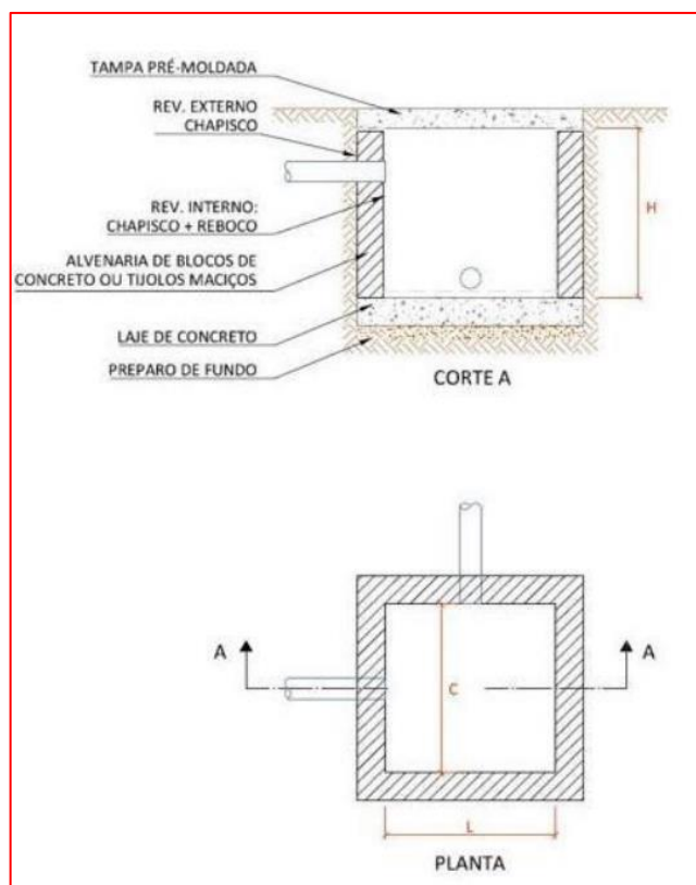
Figura 18 - Croqui de execução da caixa hidráulica – Fonte: GOOGLE
