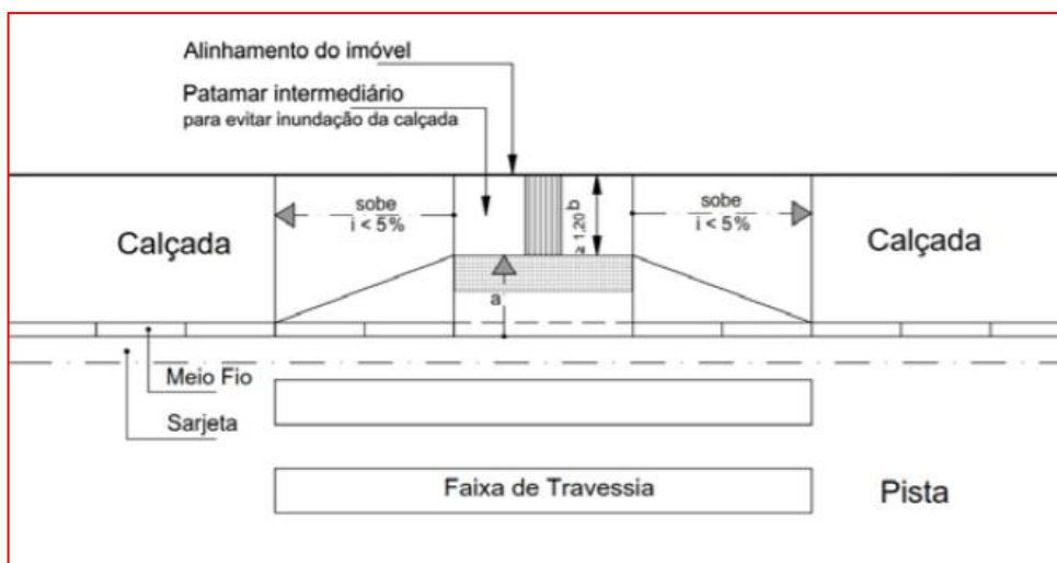
Figura 13 - Exemplo de rebaixamento de acordo com NBR 9050 – Fonte: GOOGLE
