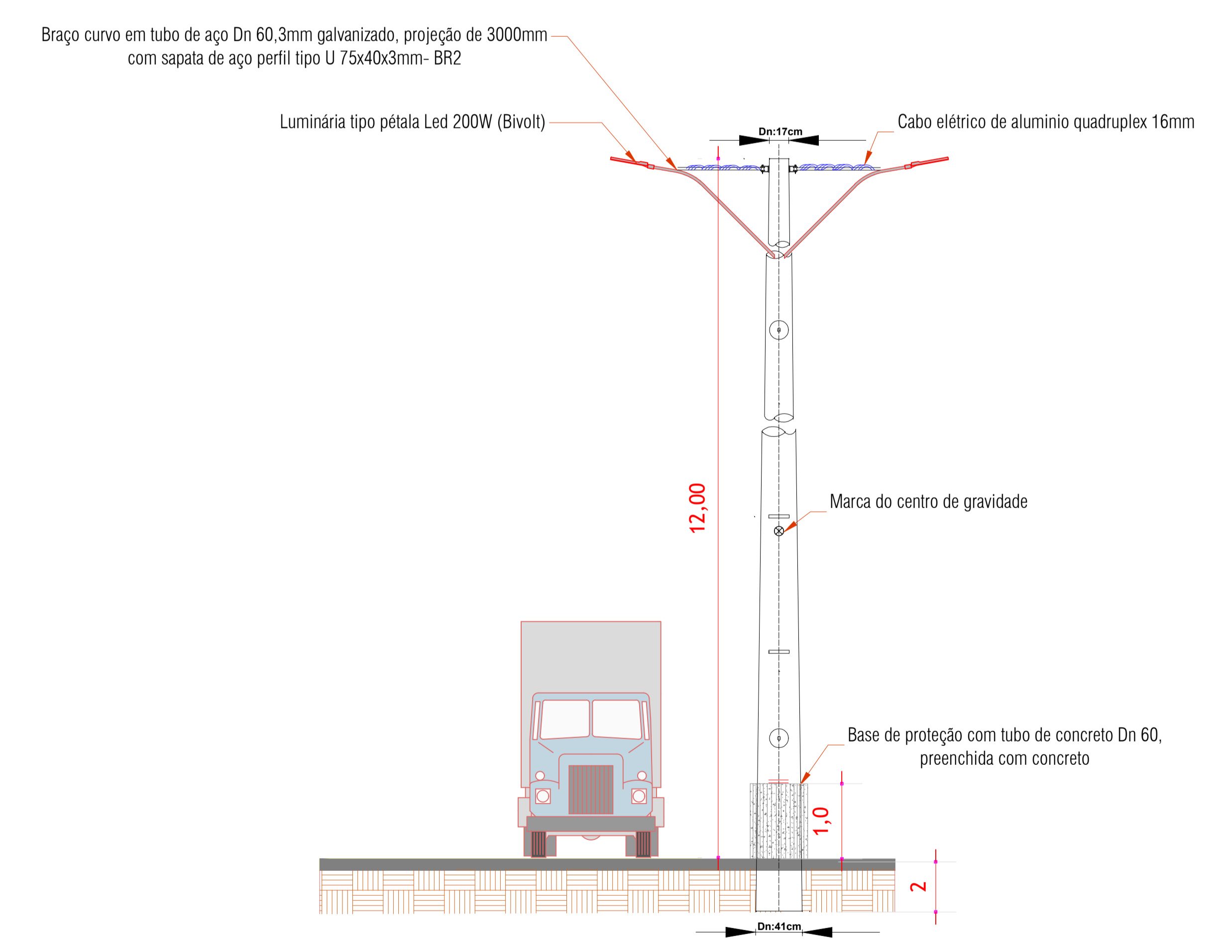
Det. Poste de Concreto Circular Escala: 1/75
