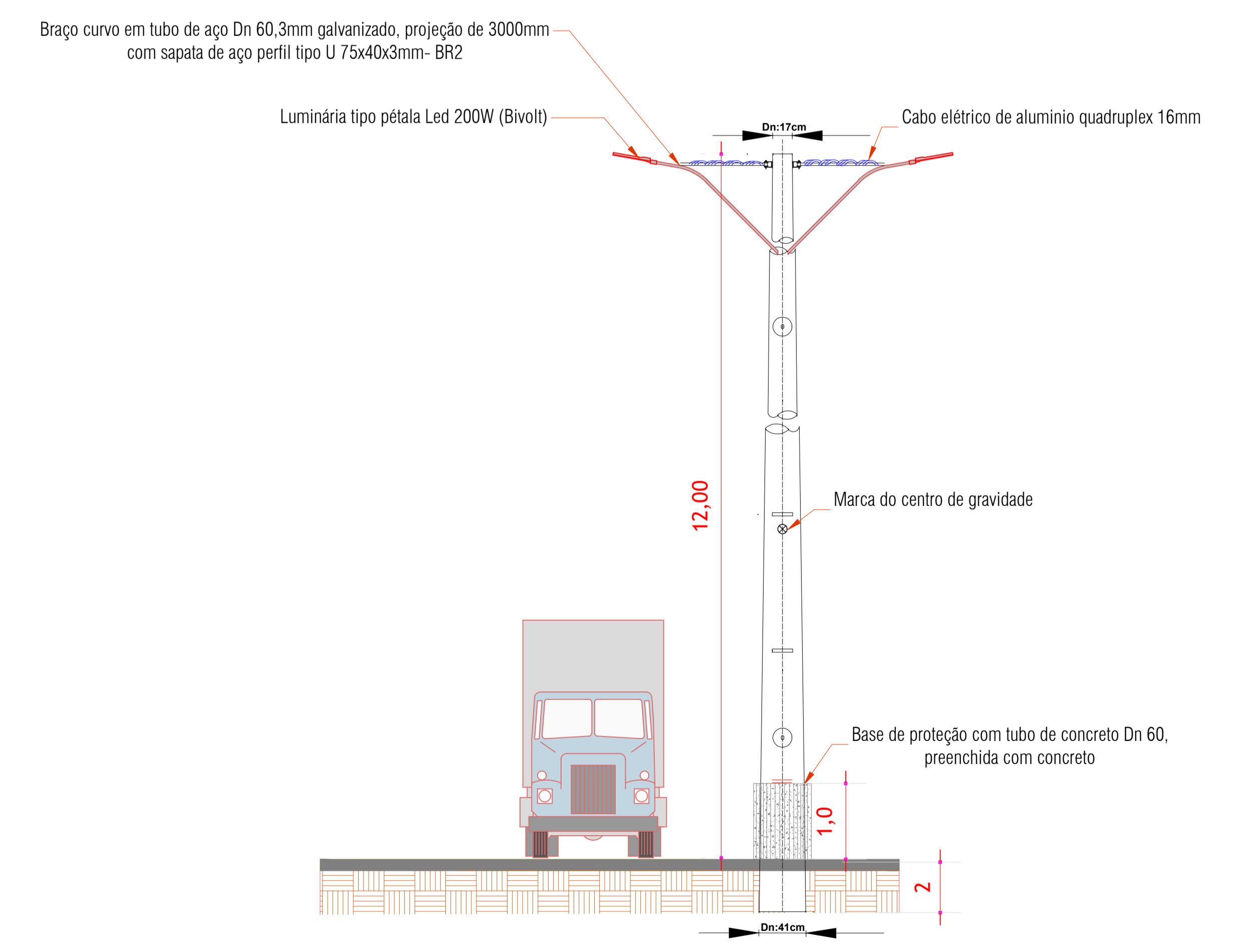
DETALHE POSTE DE CONCRETO CÔNICO ESCALA 1:75
