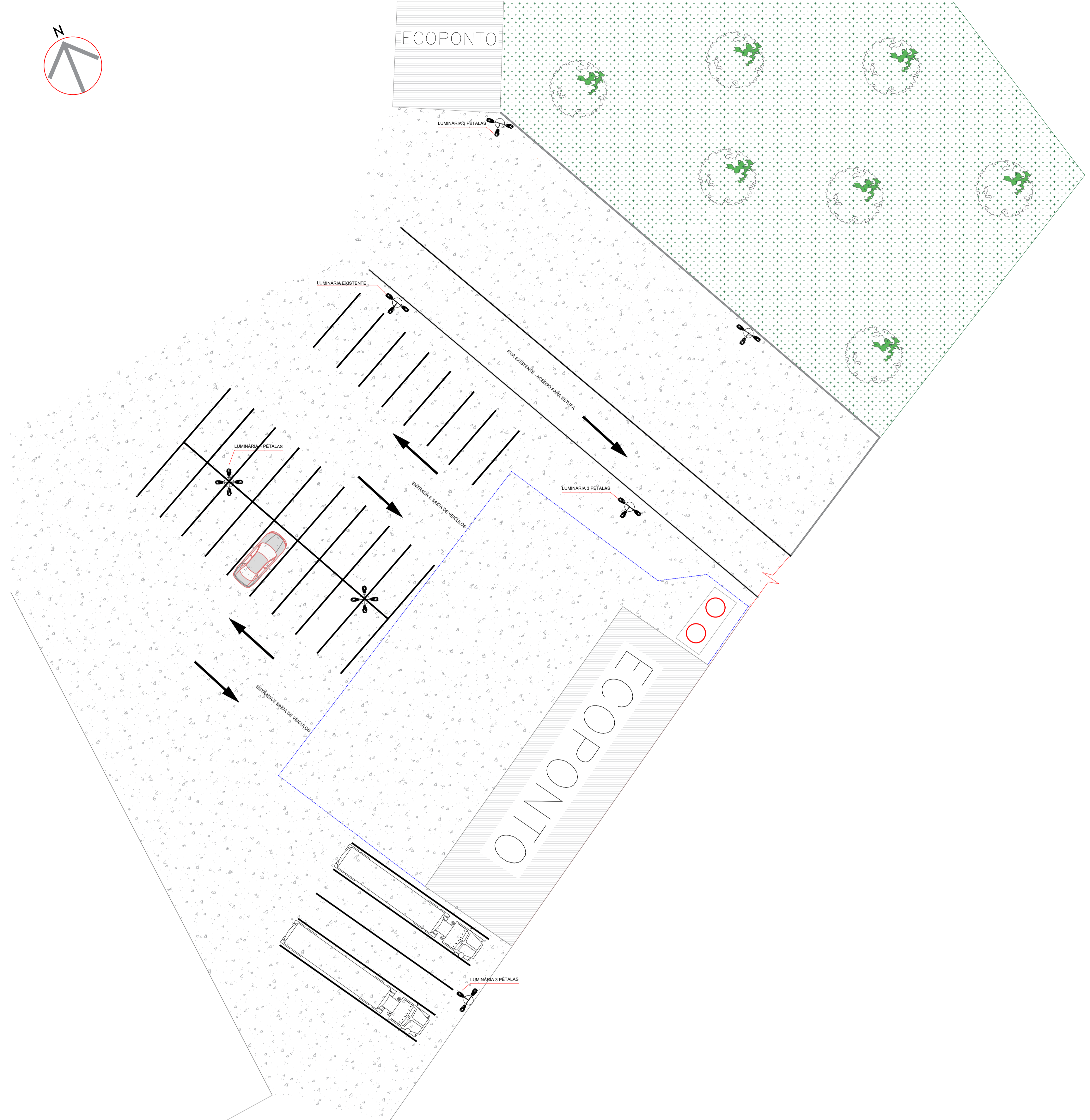
PLANTA BAIXA ILUMINAÇÃO ESTACIONAMENTO SUL Escala: 1/200
