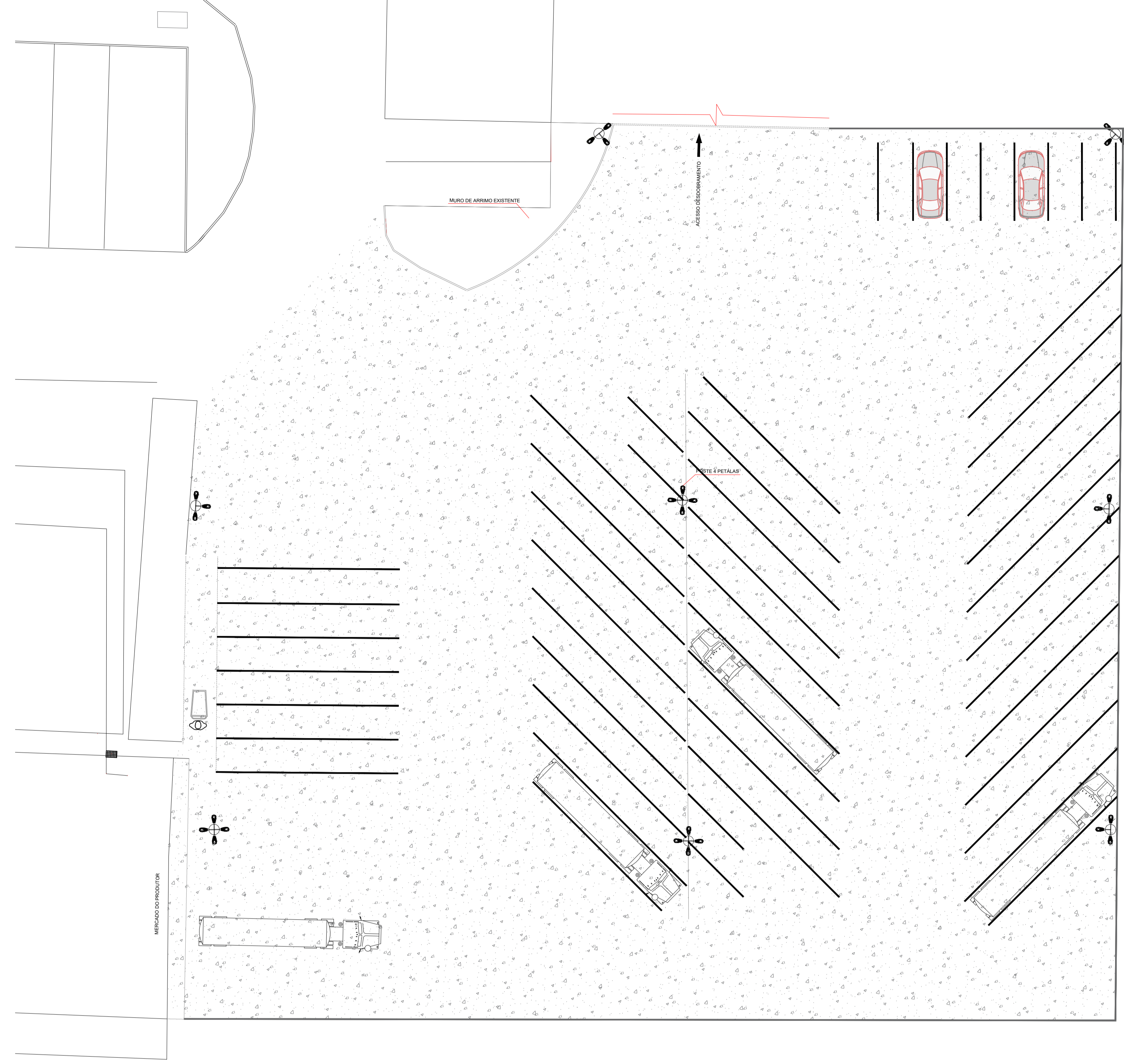
PLANTA BAIXA ILUMINAÇÃO ESTACIONAMENTO LESTE Escala: 1/200
