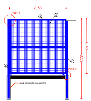
PORTÃO DE CORRER 1 FOLHA ESCALA 1:50
