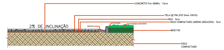
DETALHE - COMPOSIÇÃO PISO PARA ESTACIONAMENTO
