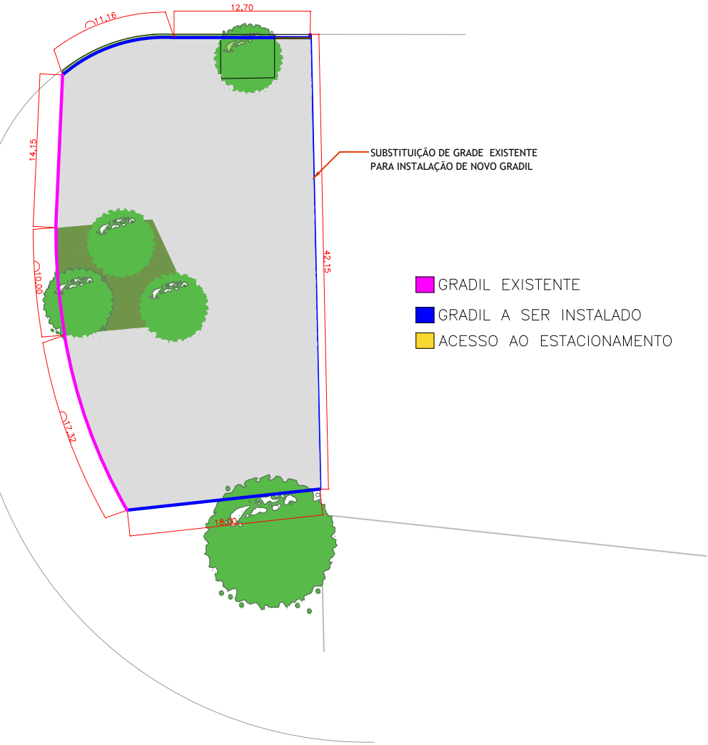
2 GRADIS ESCALA: 1/50
