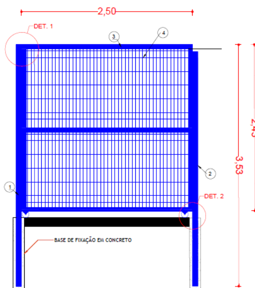
Det. Portão de Correr ESCALA 1:40
