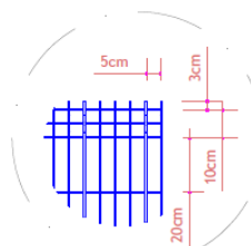
DETALHE B SEM ESCALA
