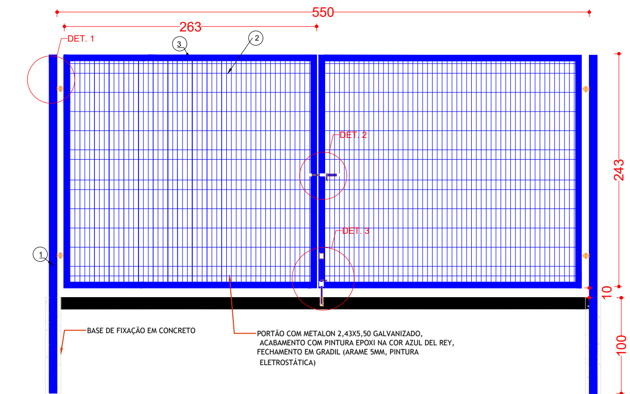
Det. Portão de Abrir ESCALA 1:40
