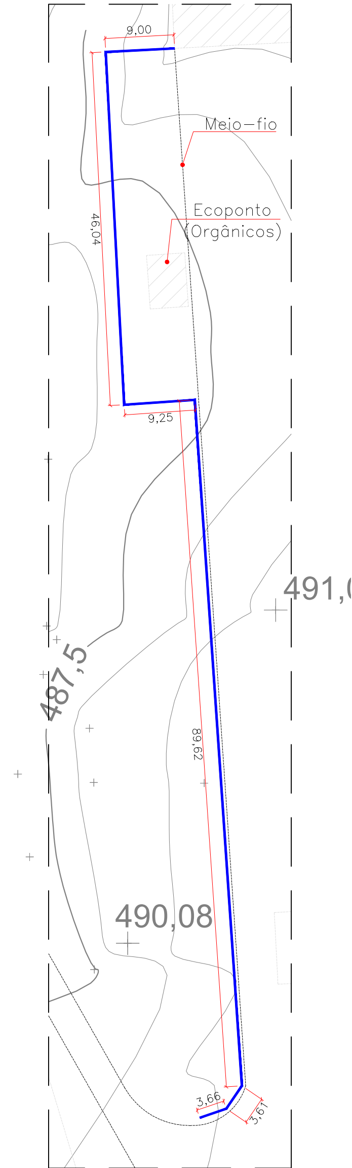
DETALHE 1 Escala 1:500
