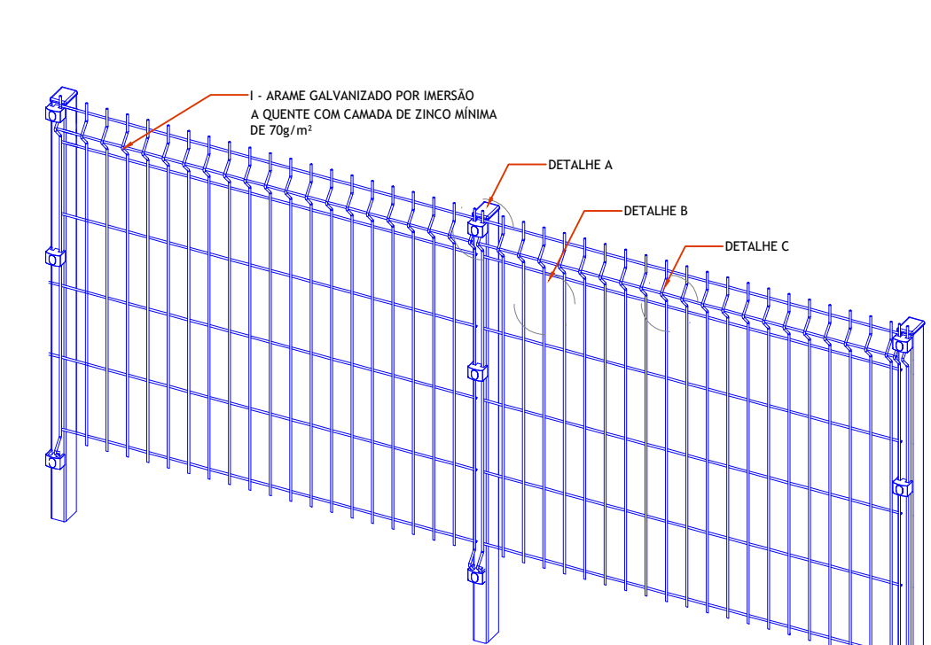
Perspectiva Gradil ESCALA 1:40
