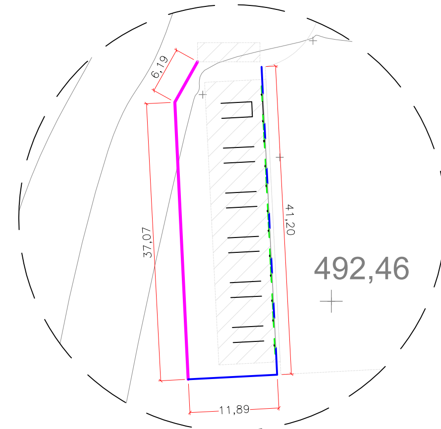
DETALHE 5 Escala 1:500
