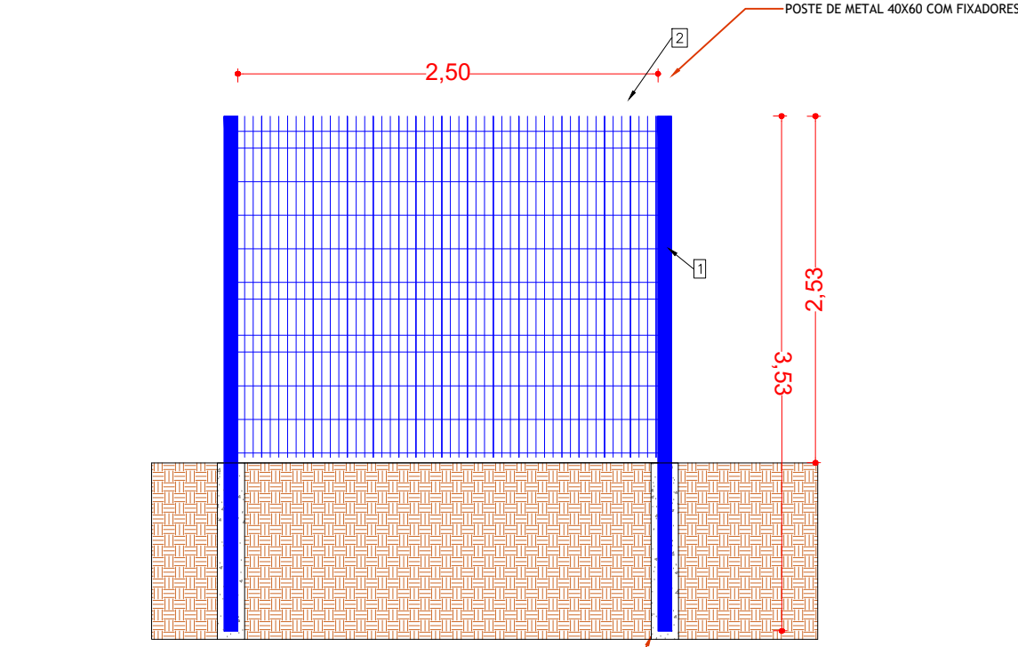
Elevação Gradil ESCALA 1:40
