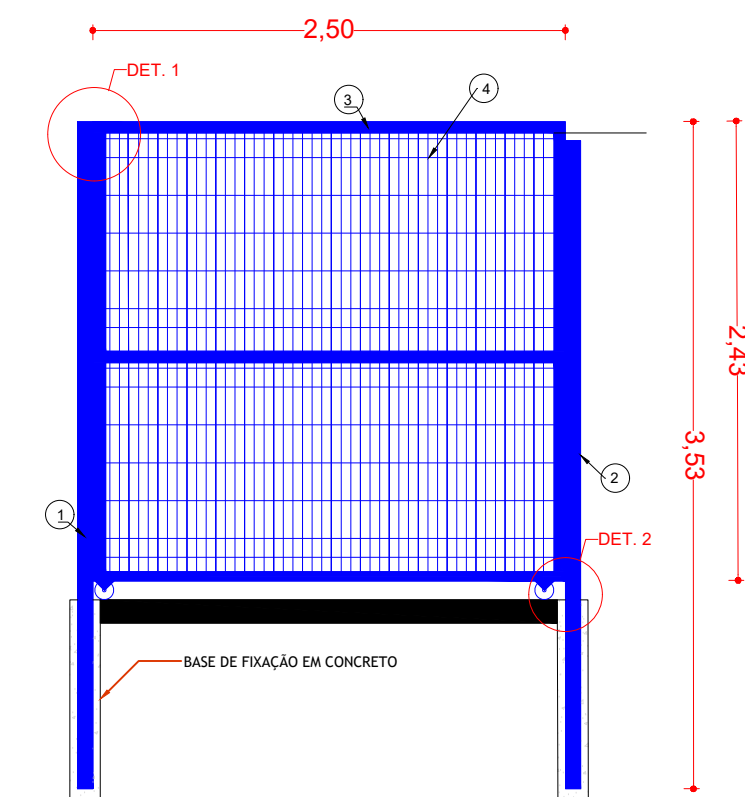
Det. Portão de Correr ESCALA 1:40
