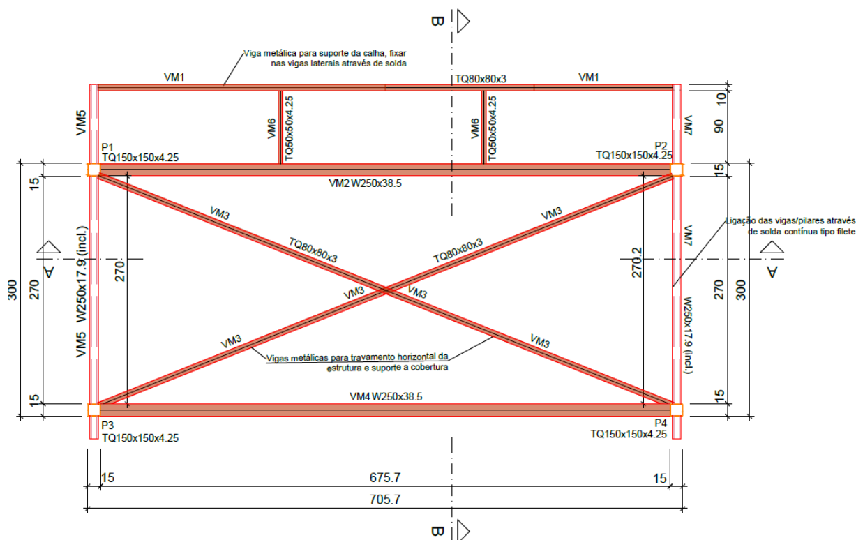
Figura 13 - Indicação dos perfis e dimensões dos elementos estruturais metálicos em projeto
