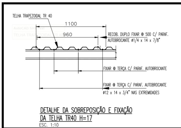
Figura 14 - Detalhamento da fixação de telhas
