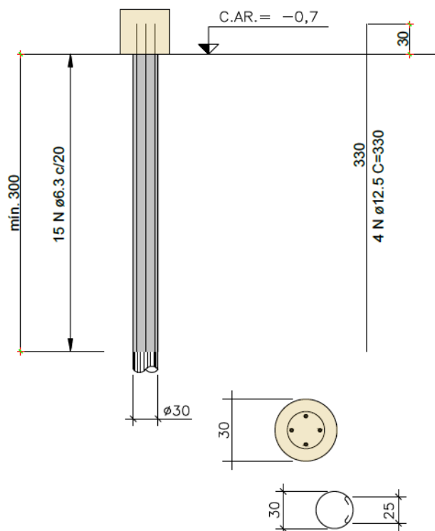
Figura 10 - Detalhamento das estacas, conforme projeto estrutural
