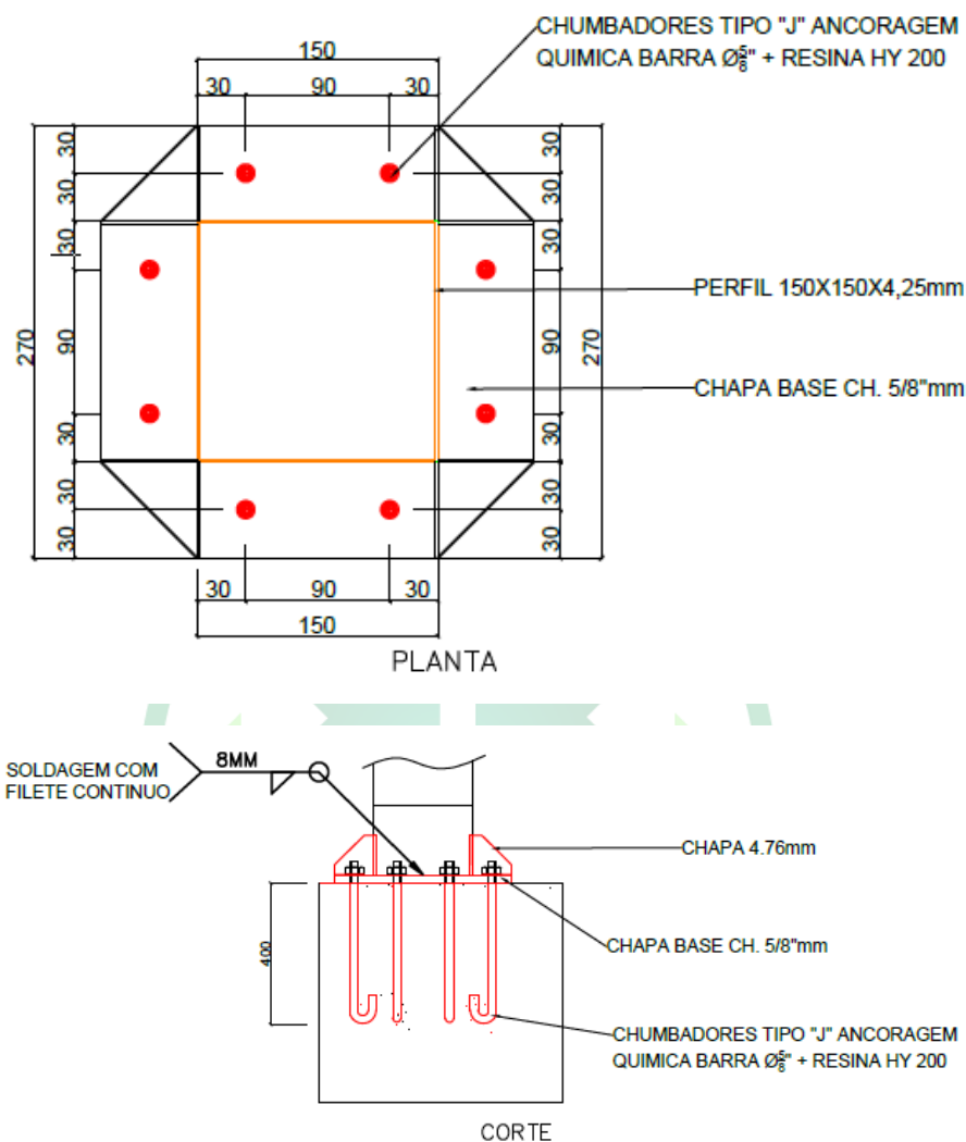
Figura 12 - Detalhe da chapa de base para os pilares
