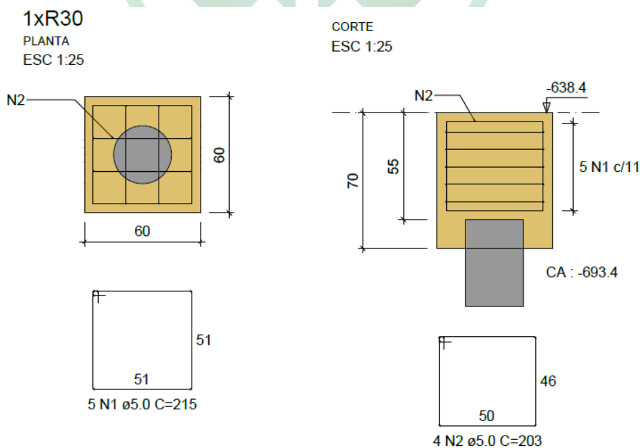
Figura 11 - Detalhamento dos blocos de concreto, conforme projeto estrutural
